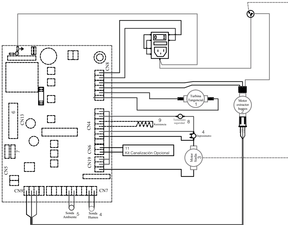
ESQUEMA ELÉCTRICO | ELECTRICAL SCHEME | SCHÉMA ÉLECTRIQUE ESQUEMA ELÉCTRICO | SCHEMA ELETRICO
